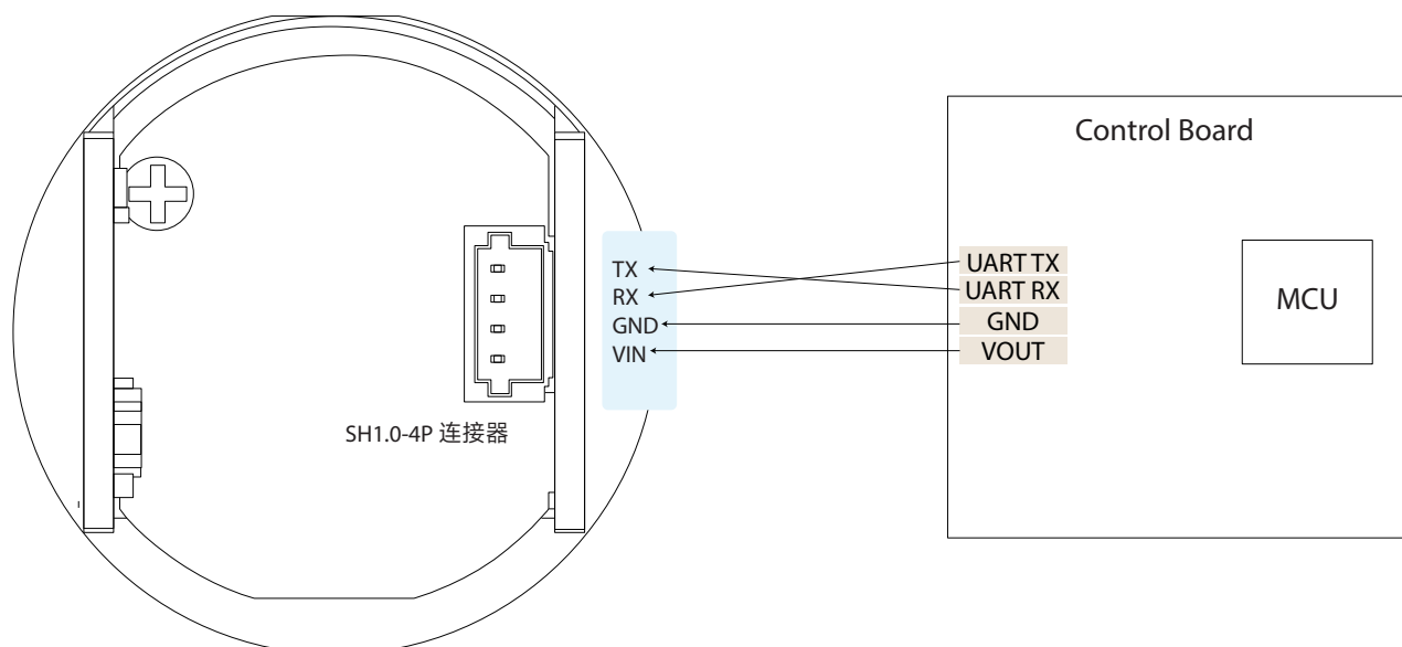
图4-1 模块引脚
