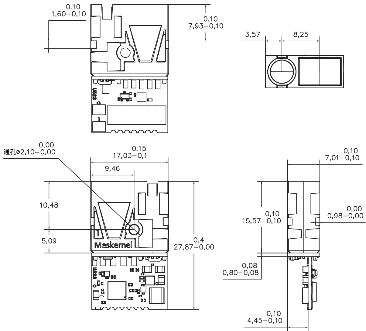
图2-1 模块概览图
