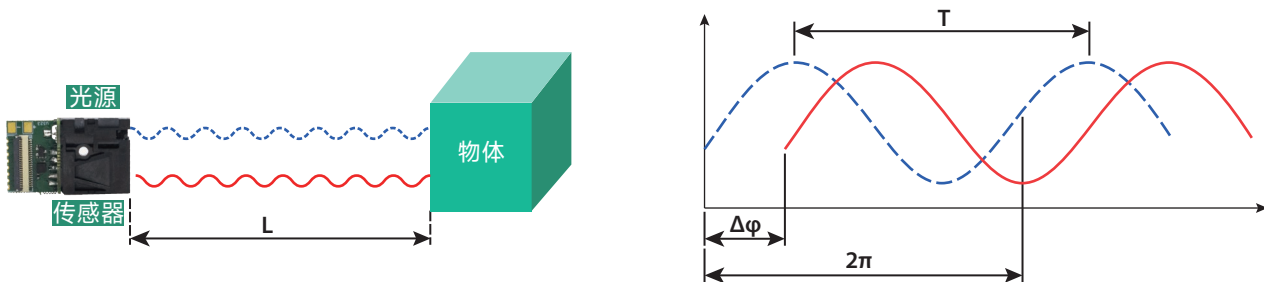
图1-1 激光模块基本原理图
