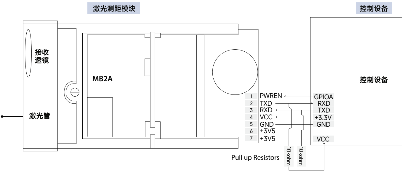
图4-1 模块引脚布局及推荐连线
