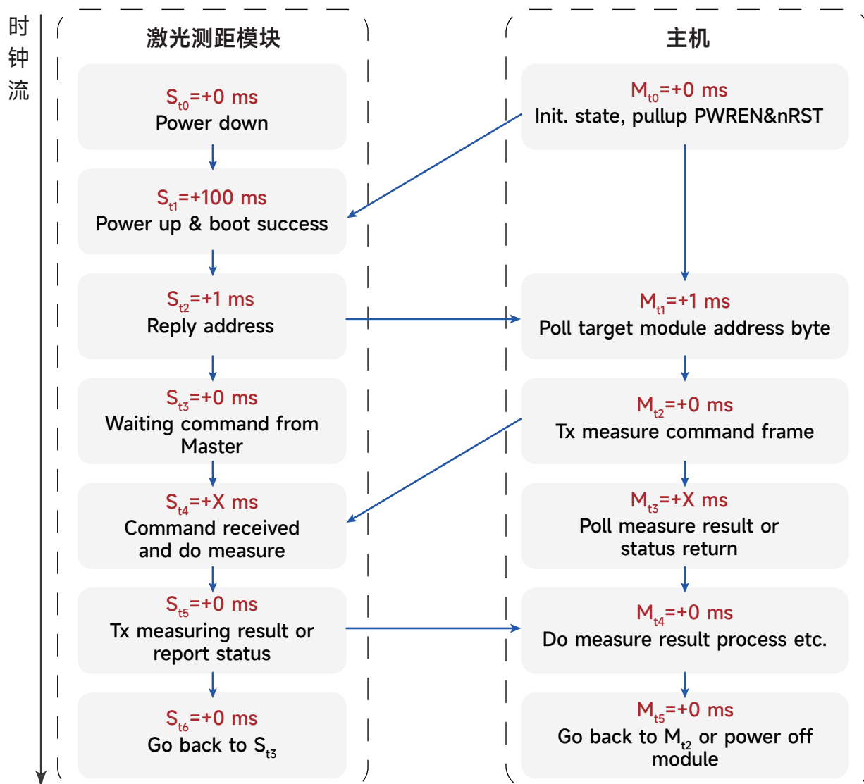
图10-1 模块通信时间线
