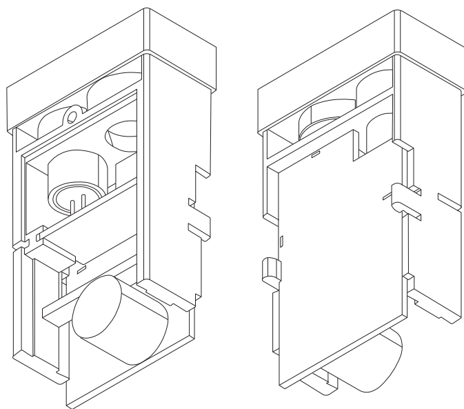
图2-1 模块概览图
