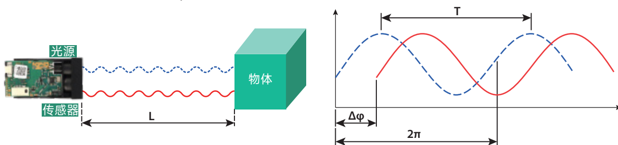
图1-1 激光模块基本原理图
