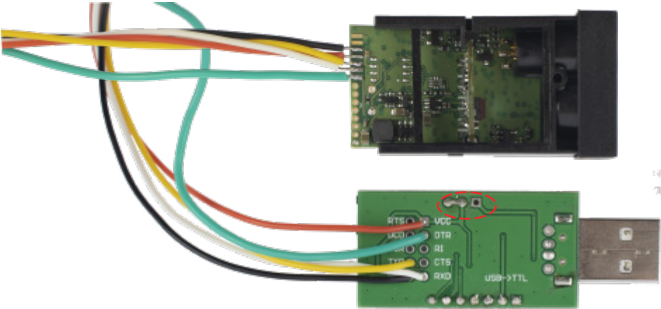
图5-2 焊接
